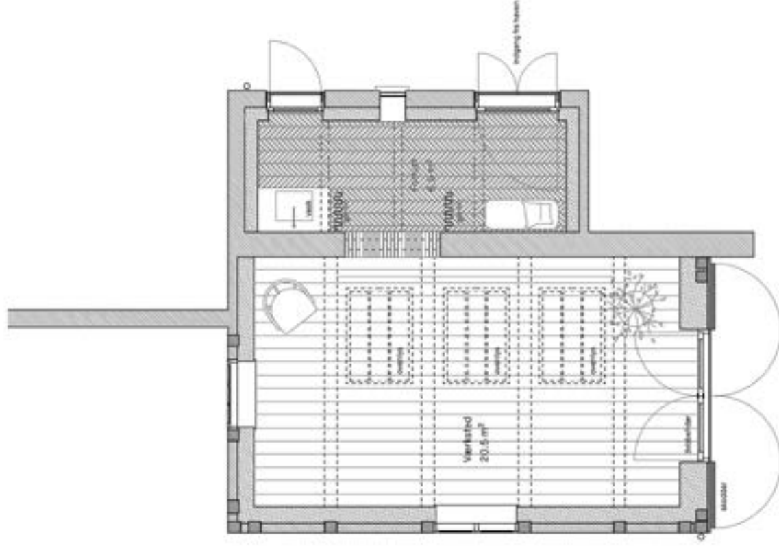
Plan - Annekset. Fremtidige forhold - mst 1:50
